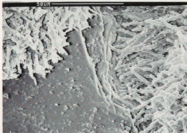
Figura 5: Imatge que presenten al microscopi electrònic els filaments de líquens que colonitzen la pedra, i els petits cristalls d'oxalats de calci associats a l'activitat d'aquests organismes.
