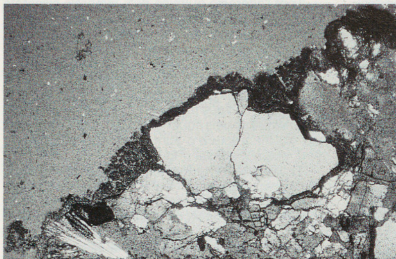
Figura 6: Visió al microscopi òptic de la pàtina de matèria orgànica que recobreix parcialment la pedra i que produeix la disgregació de la pedra en penetrar, com s'observa a la fotografia, per les interfases minerals. A la banda inferior esquerra de la fotografia s'observa també l'expansió que presenten els plans d'exfoliació de les biotites superficials en patir hidròlisi.
